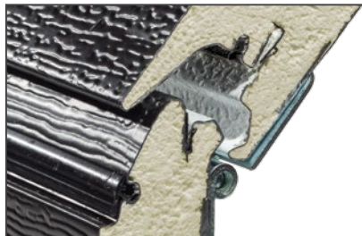
Garniture double entre chaque section qui assure un ajustement précis et réduit l'infiltration d'air.
